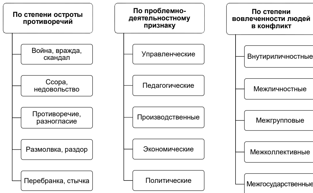
Рисунок 2 – Классификация конфликтов
